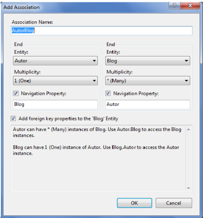
Figura 2.61.- Creación de una asociación en Model First
