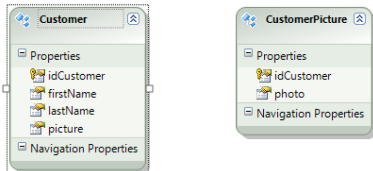
Figura 2.31.- La entidad CustomerPicture con las entidades pegadas
