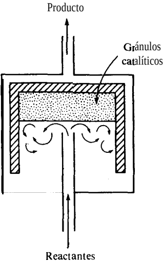
Fig. II-10 Reactor para un solo gránulo catalítico plano.
