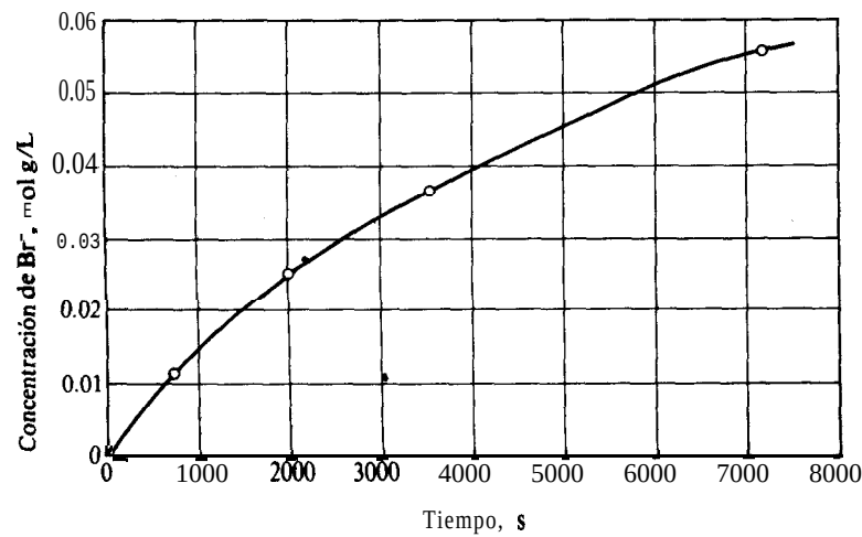
Fig. 2-4. Concentración en función del tiempo para la reacción entre (CH_3)_3N y CH_3CH_2CH_2Br .
