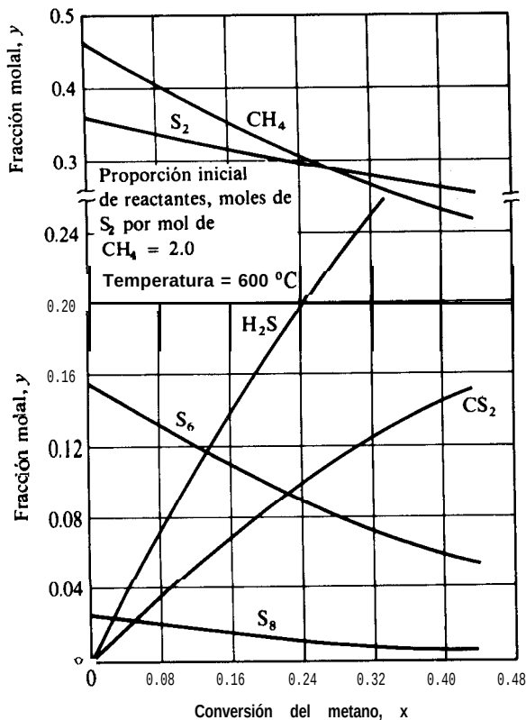
Fig.4-5 Composici3n de la mezcla reaccionante en funci3n de la conversi3n para la sulfuraci3n del metano.
