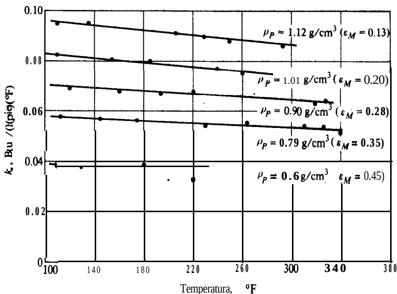
Fig. 11-4 Conductividad térmica efectiva de gránulos catalíticos de alúmina (boehmita) a 10-25 \mu de Hg de presión.
