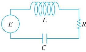
FIGURA 5.1.15 Circuito LRC en serie.
