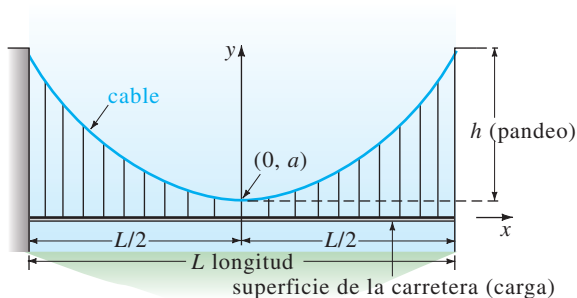
FIGURA 2.2.5 Forma de un cable del problema 49.
