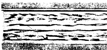
Figura 1.2 Flujo en la zona crítica, entre las zonas laminar y de transición A la velocidad crítica los filamentos comienzan a romperse, indicando que el flujo comienza a ser turbulento.
