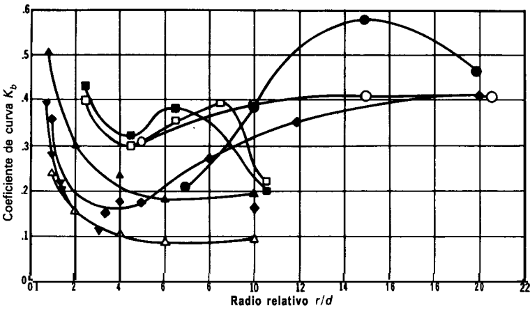
Figura 2-15. Coeficientes de curva deducidos por varios investigadores (Beij 21 ). Tomado de "Pressure losses for Fluid Flow in 90° Pipe Bends", de K.H. Beij. Por cortesía del Journal of Research of National Bureau of Standards
