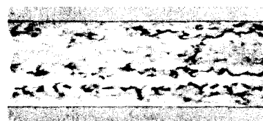
Figura 1.3 Flujo turbulento Esta fotografía muestra cómo la turbulencia en la corriente dispersa completamente los filamentos coloreados a poca distancia del punto de introducción.
