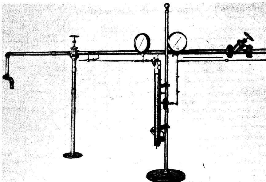
Figura 2-10 Sistema de tuberías para prueba de válvulas de globo en Y, de acero, de 0.5 pulgadas (50 mm).
