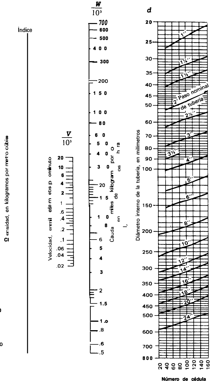
Nomograma VI-a
