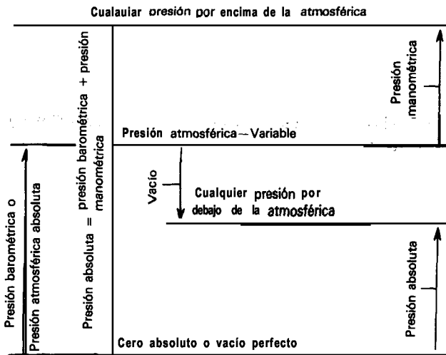
Figura 1-5 Relación entre las presiones manométrica y absoluta
