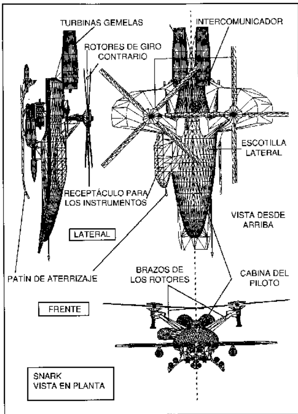
SNARK HELICÓPTERO DE ATAQUE DE ROTORES GEMELOS
