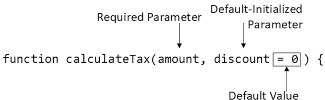
Figure 8-2. Defining a default parameter value
