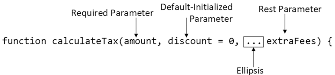
Figure 8-3. Defining a rest parameter
